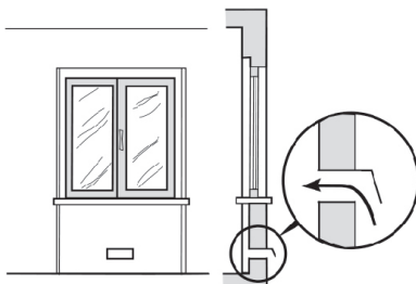
Пример обеспечения притока воздуха
