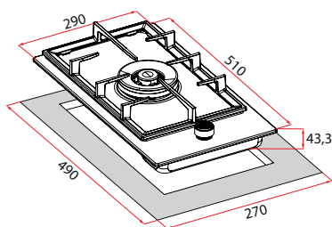
HGM 31404
