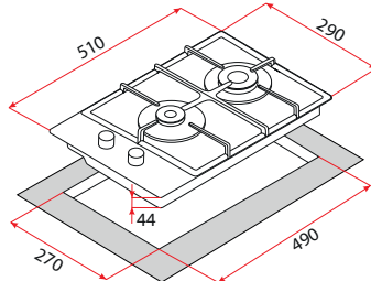
HGM 31424
