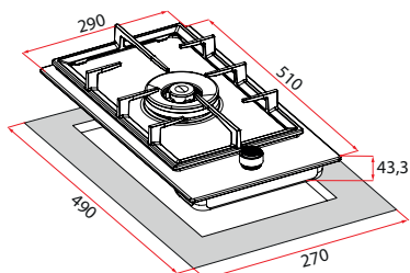
HGM 31404
