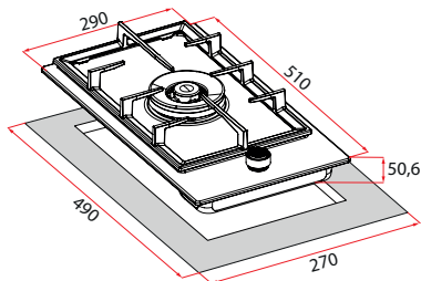
HGG 31404
